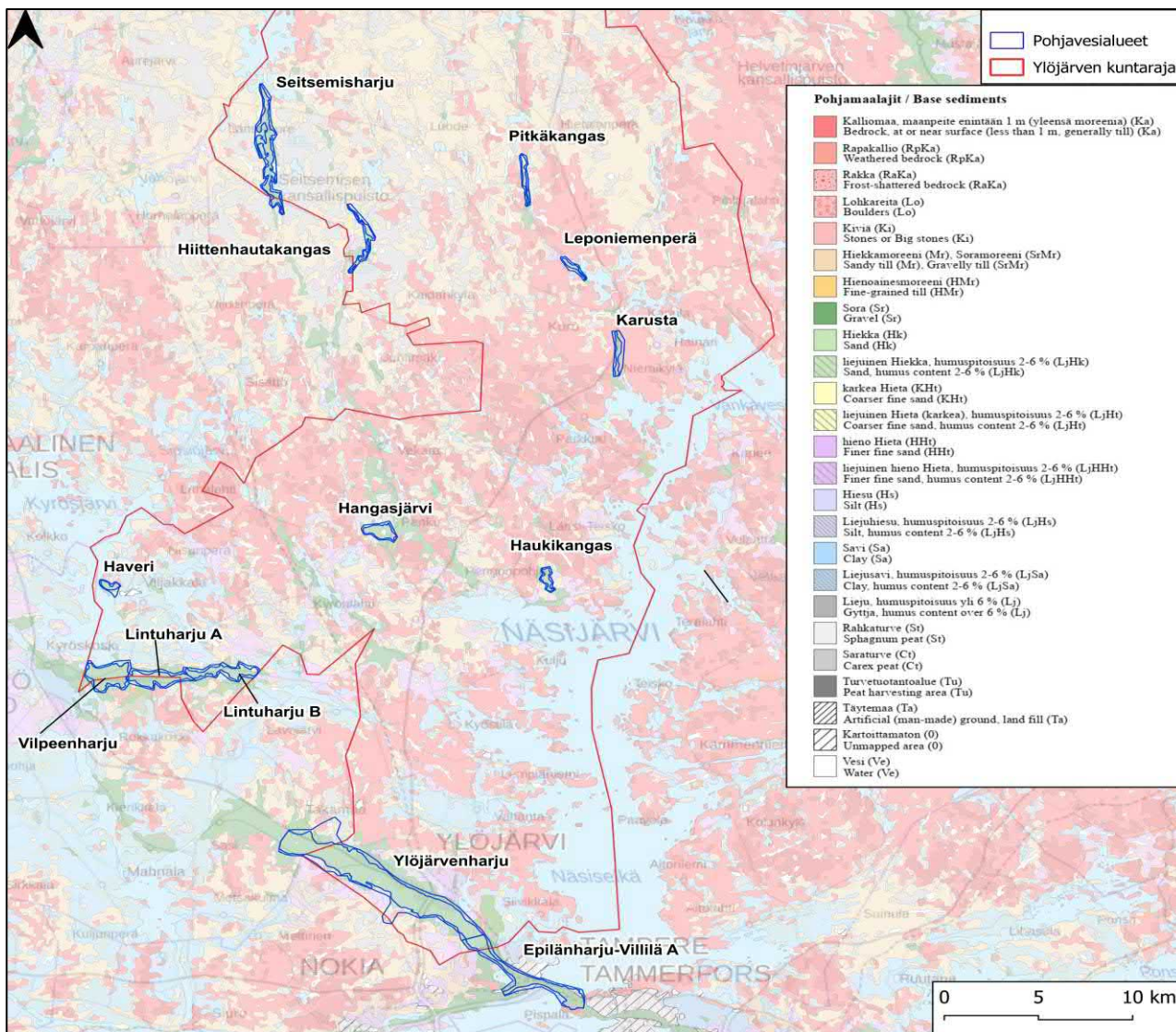
Kuva 3. Maaperäkarta (200k) Ylöjärven alueella (GTK 2002-2009).
