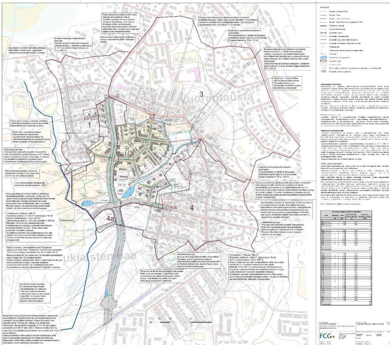
Kuva 19. Hulevesien hallinnan yleissuunnitelma, FCG 19.4.2023.
